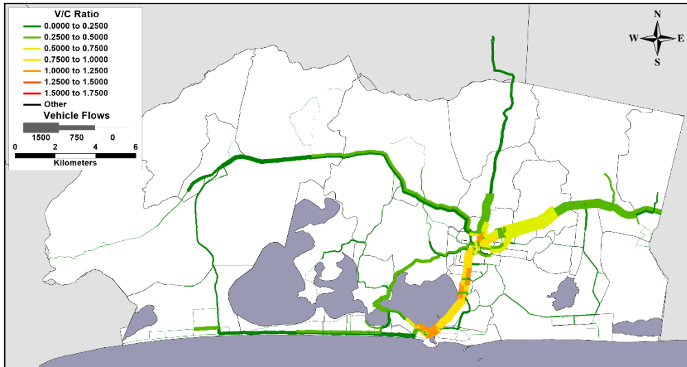
Figura 83: Carregamento da rede – cenário 1 (nada a fazer, tendência Acelerado), ano 2024
