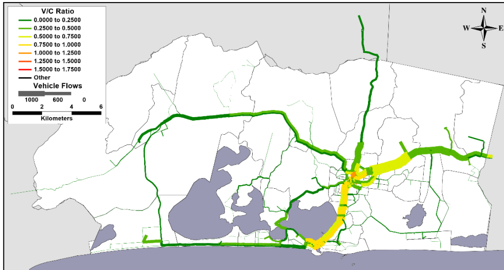
Figura 87: Carregamento da rede – cenário 3 (projetos, tendência moderada), ano 2027
