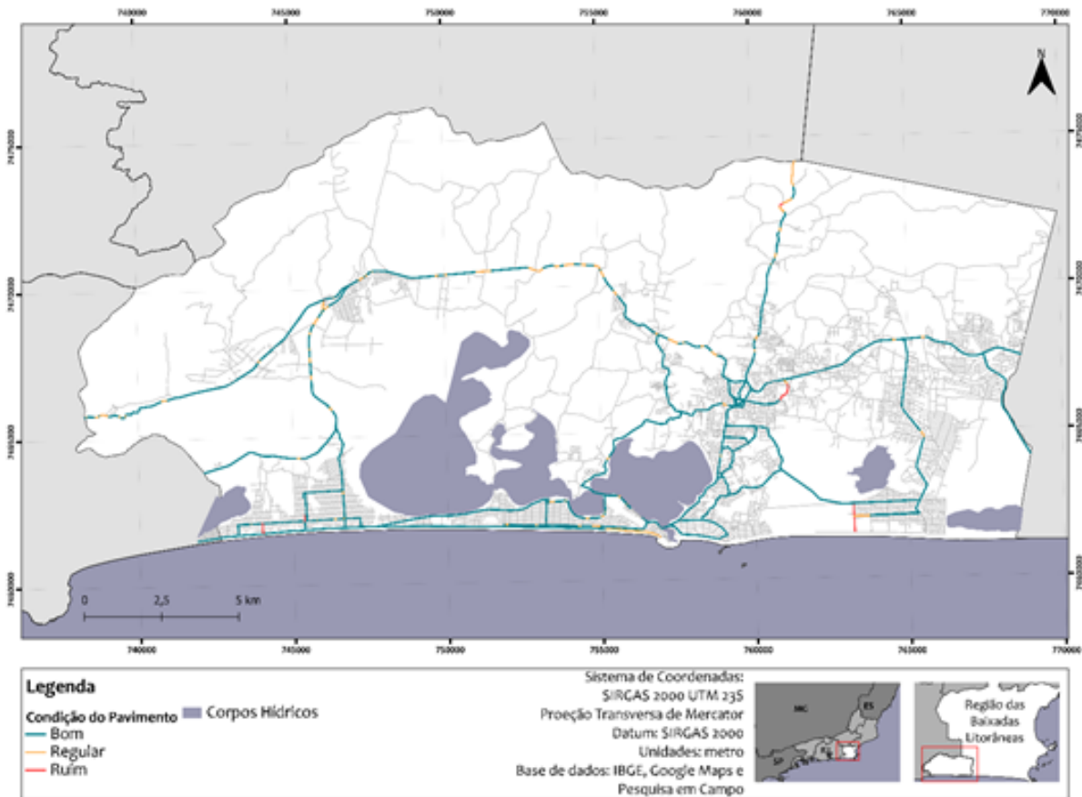
Figura 30: Condição do pavimento
