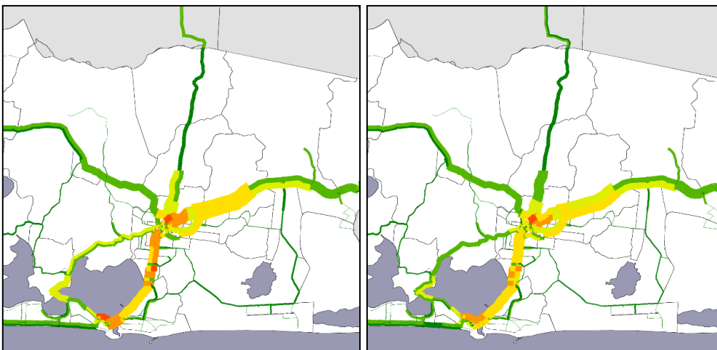
Figura 97: Carregamento da rede - comparação Cenários 2 e 4, ano 2032
