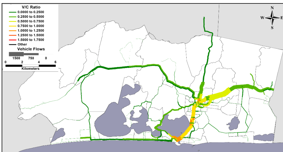
Figura 89: Carregamento da rede – cenário 4 (projetos, tendência Acelerado), ano 2024
