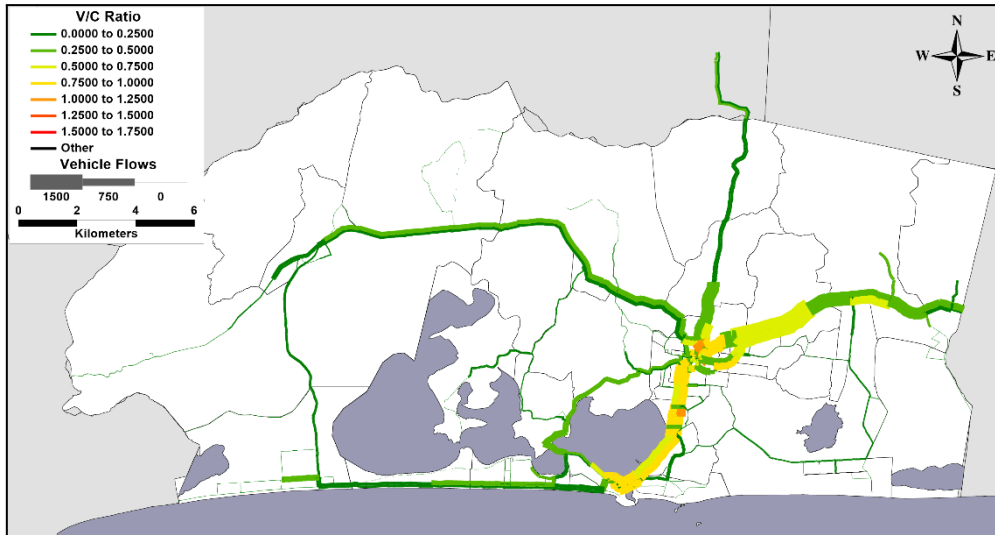
Figura 90: Carregamento da rede – cenário 4 (projetos, tendência Acelerado), ano 2027
