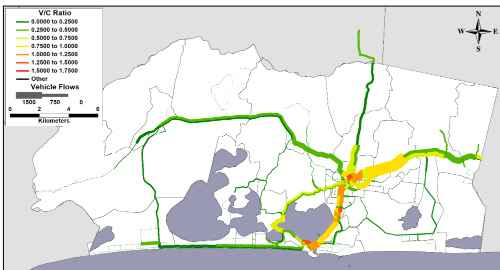
Figura 85: Carregamento da rede – cenário 1 (nada a fazer, tendência Acelerado), ano 2032
