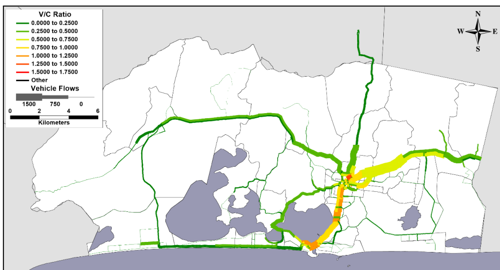
Figura 82: Carregamento da rede – cenário 1 (nada a fazer, tendência moderada), ano 2032
