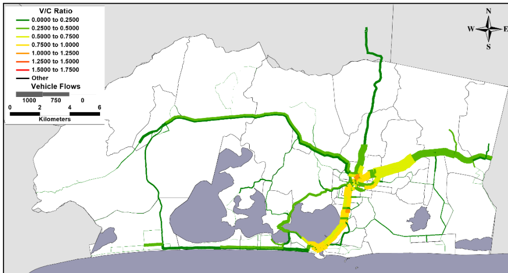
Figura 88: Carregamento da rede – cenário 3 (projetos, tendência moderada), ano 2032
