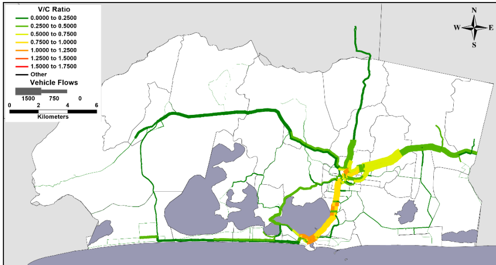
Figura 80: Carregamento da rede – cenário 1 (nada a fazer, tendência moderada), ano 2024
