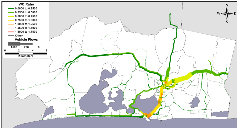
Figura 81: Carregamento da rede – cenário 1 (nada a fazer, tendência moderada), ano 2027
