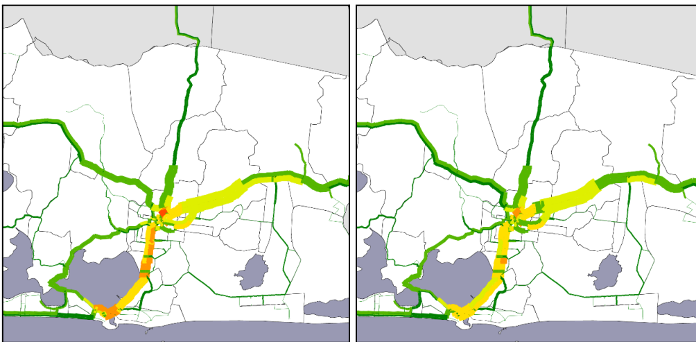
Figura 96: Carregamento da rede - comparação Cenários 2 e 4, ano 2027
