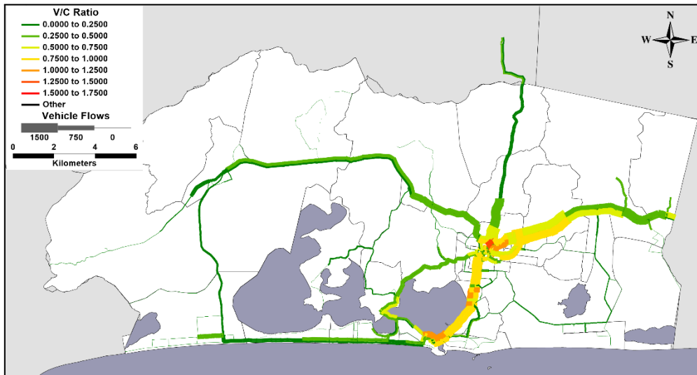
Figura 91: Carregamento da rede – cenário 4 (projetos, tendência Acelerado), ano 2032
