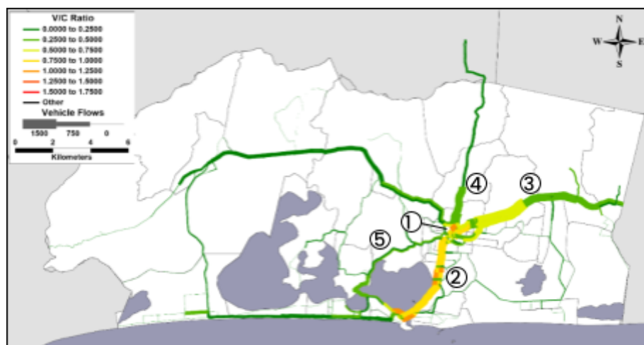
Figura 79: Carregamento da rede – ano base
