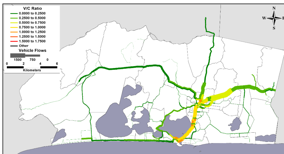
Figura 86: Carregamento da rede – cenário 3 (projetos, tendência moderada), ano 2024
