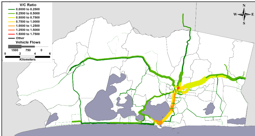
Figura 84: Carregamento da rede – cenário 1 (nada a fazer, tendência Acelerado), ano 2027
