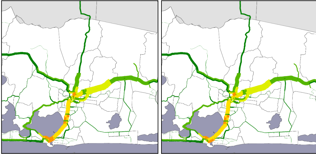
Figura 92: Carregamento da rede - comparação Cenários 1 e 3, ano 2024
